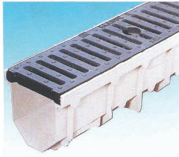
Stigerist i støbejern belastningsklasse C250
